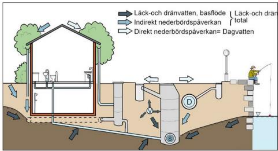
Figur 7. Källor till tillskottsvatten. Från (Svenskt Vatten utveckling, 2020).
